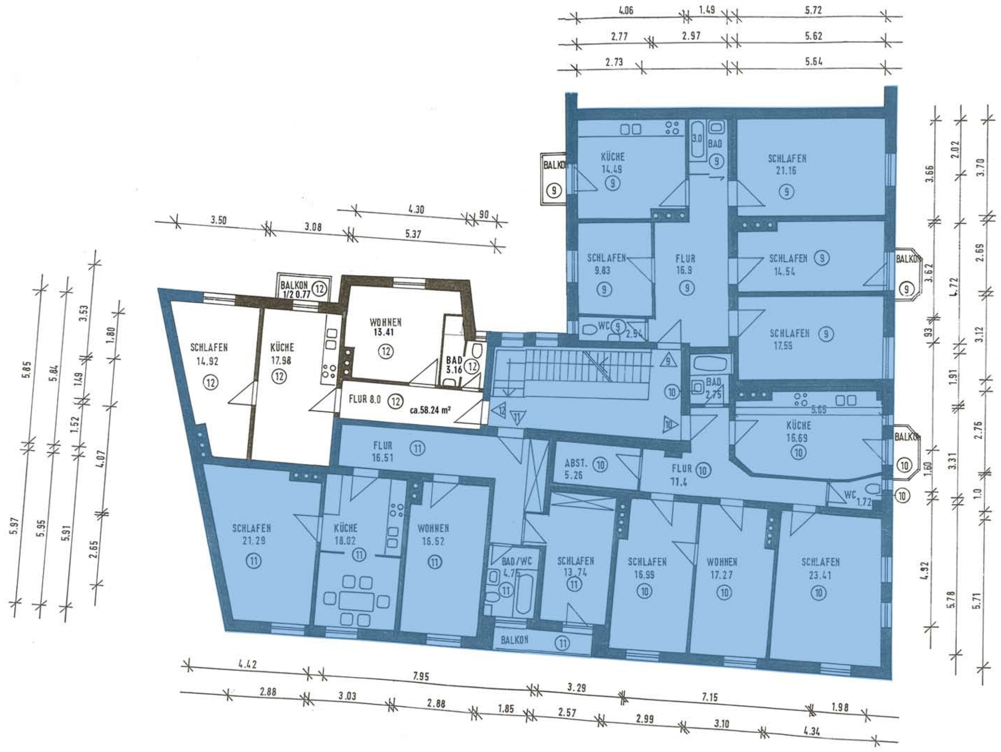
2.OBERGESCHOSS_Arnulfstrasse 140
