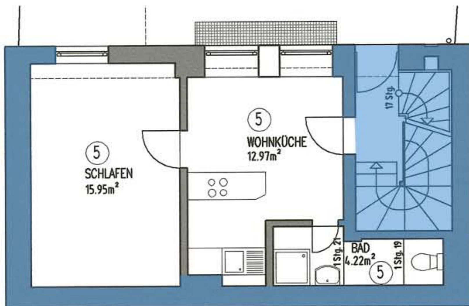
1. OBERGESCHOSS RÜCKGEBÄUDE
