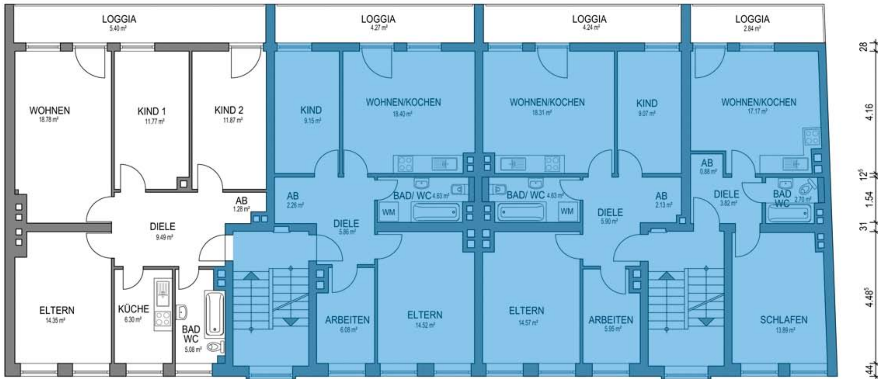
Wohnung 04 84.32 m 2
