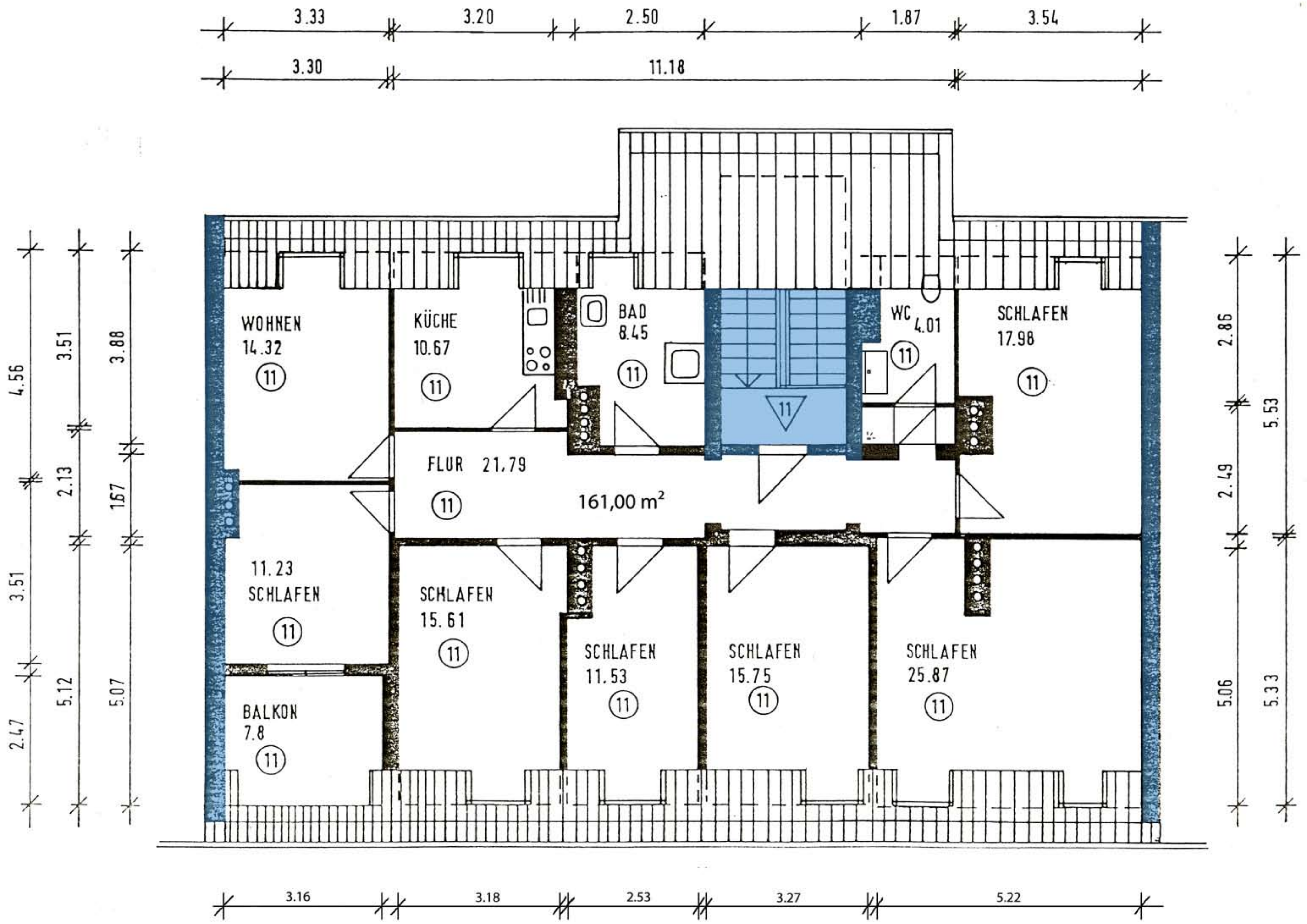
DACHGESCHOSS_Lindwurmstrasse 40
