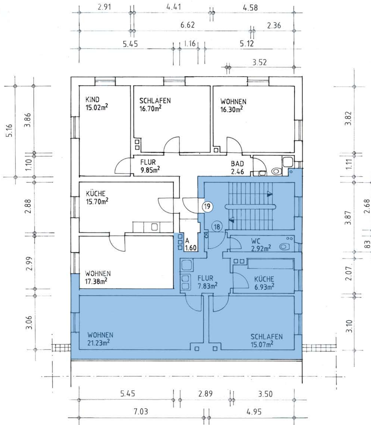
1.OBERGESCHOSS_Schleißheimerstrasse 88_Rückgebäude
