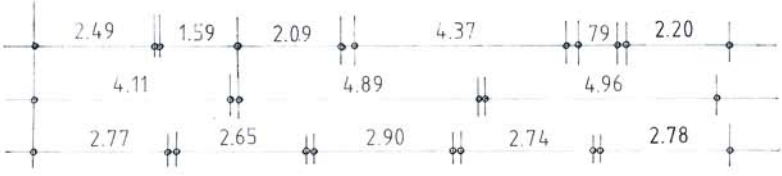
1.OBERGESCHOSS_Schleißheimerstrasse 88_Vordergebäude
