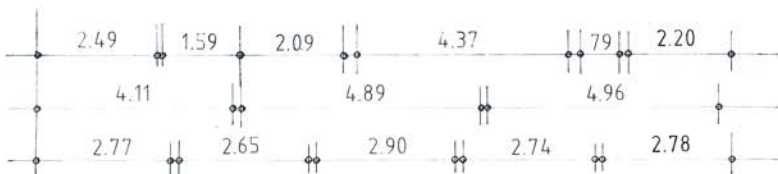
1.OBERGESCHOSS_Schleißheimerstrasse 88_Vordergebäude
