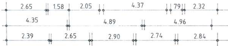
3.OBERGESCHOSS_Schleißheimerstrasse 88_Vordergebäude
