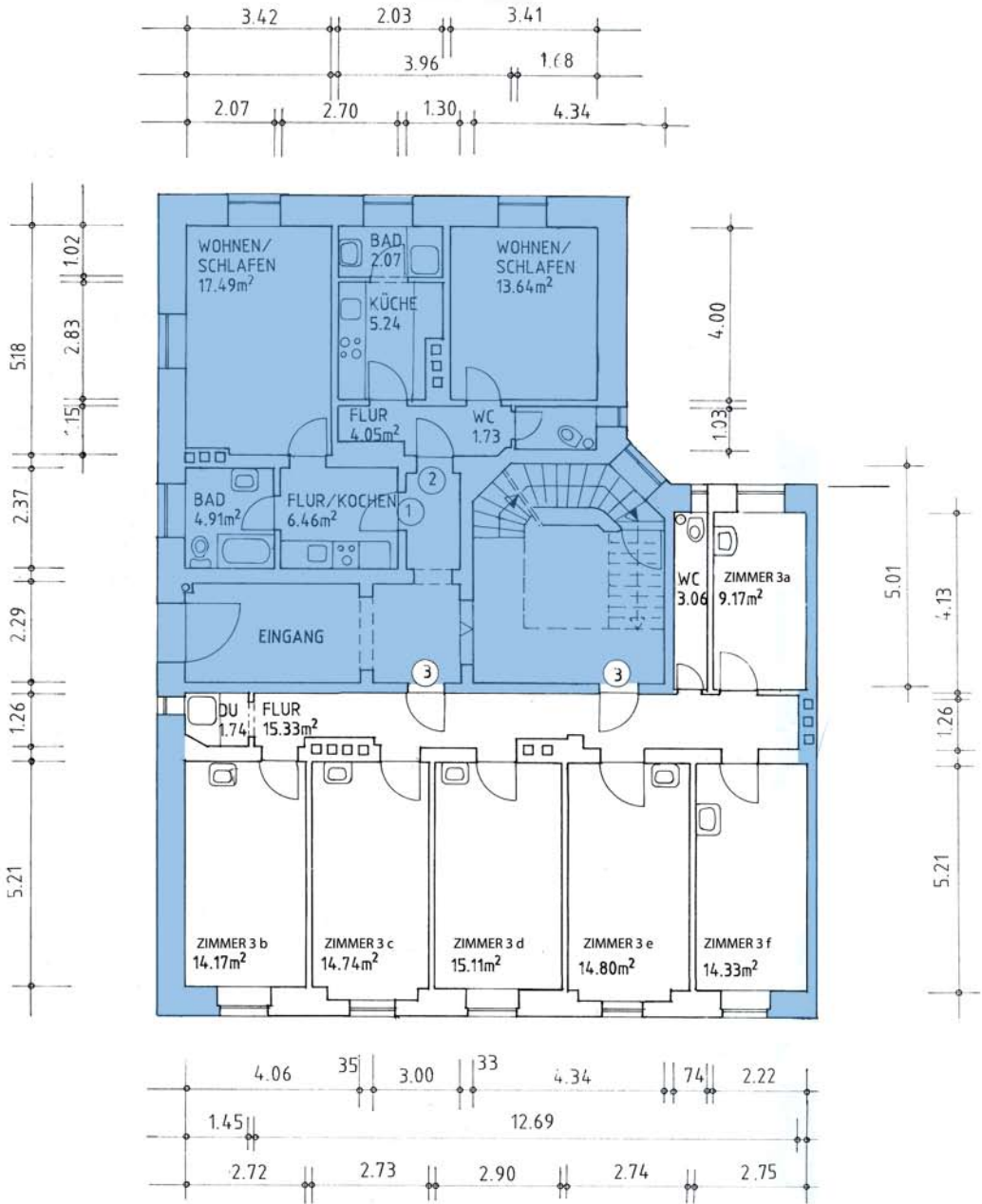
ERDGESCHOSS_Schleißheimerstrasse 88_Vordergebäude
